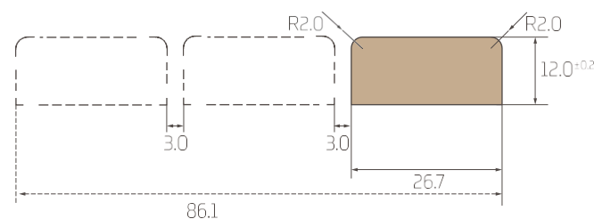
Lamela ■ 12x27
